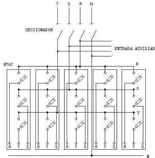
Fig. 1a: CBT-EAS con 5 salidas
