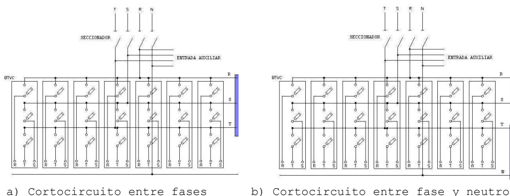
Figura 5: Disposición de las barras para ensayo de cortocircuito
