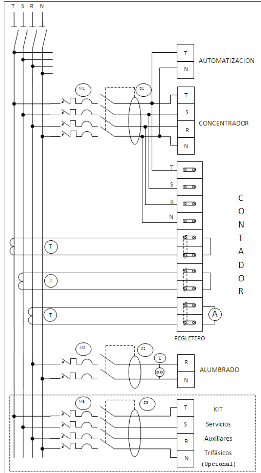
Fig. 3: Esquema del control y alimentación equipos de telegestión
