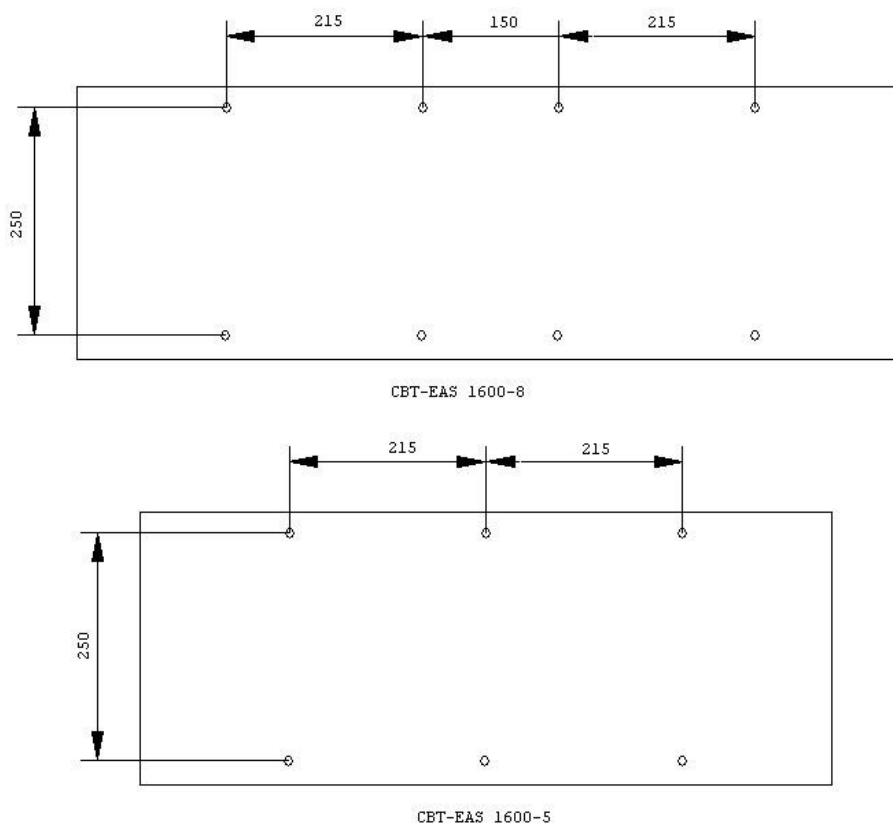
Fig. 4: Dimensiones del anclaje (mm)
